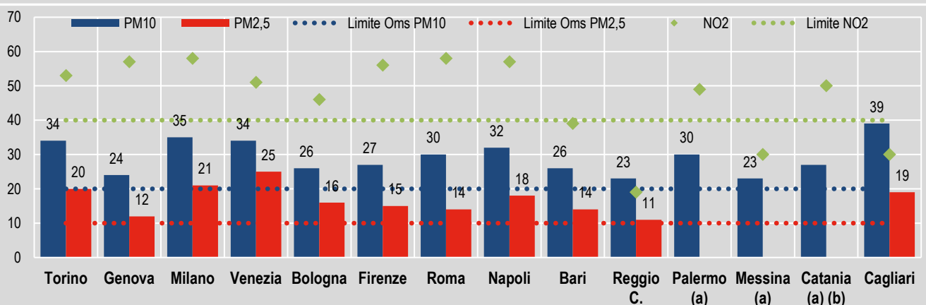
FIGURA 13. CONCENTRAZIONI MEDIE ANNUE DI PM 10 , PM 2,5 E NO 2 NEI CAPOLUOGHI METROPOLITANI. Anno 2019, valori massimi misurati tra tutte le centraline di monitoraggio in µm 3
